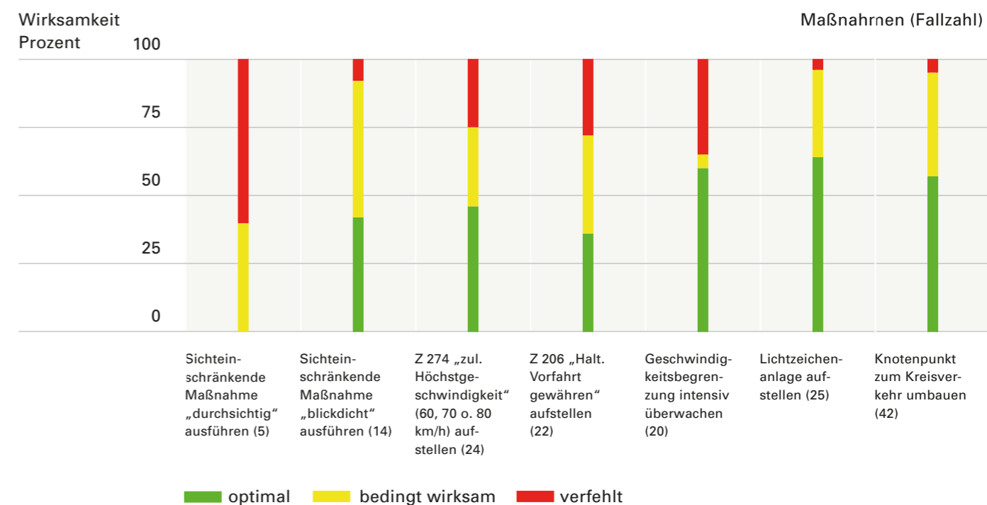
» Abb. 24 Wirksamkeit von Maßnahmen an unfallauffälligen verkehrszeichengeregelten Knotenpunkten außerorts in Bayern mit hauptsächlich Vorfahrtsverletzungen
