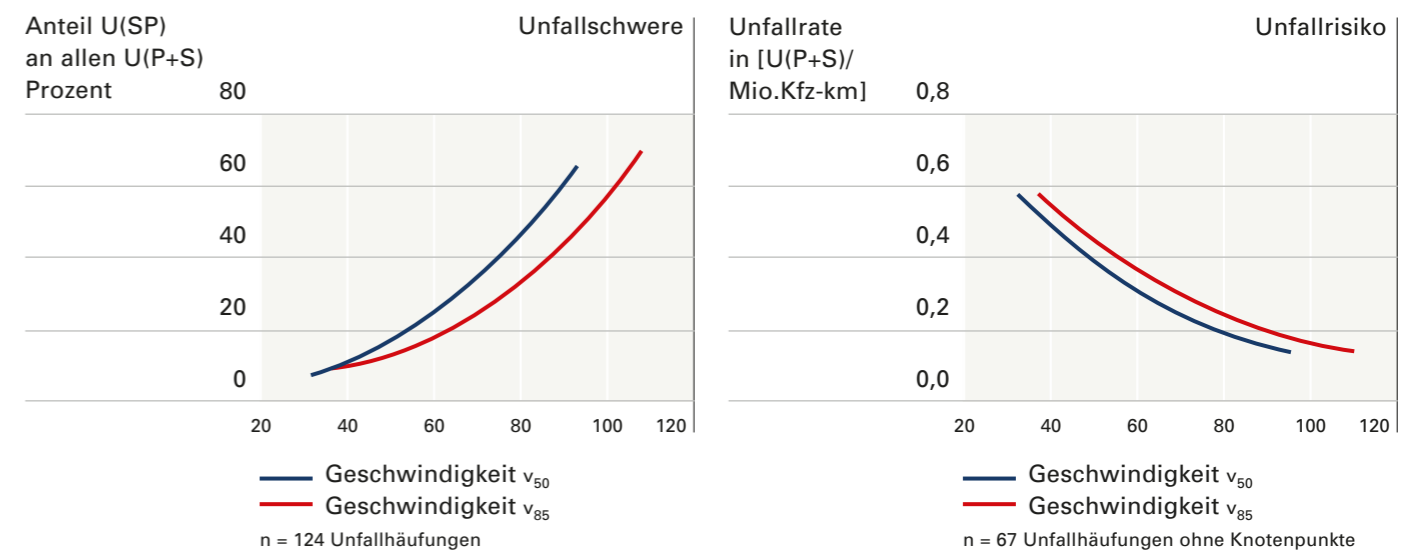
» Abb. 21 Unfallschwere und Unfallrisiko nach Geschwindigkeiten v_{50} und v_{85} der untersuchten Unfallhäufungen auf Bundes-, Staats- und Kreisstraßen außerorts
